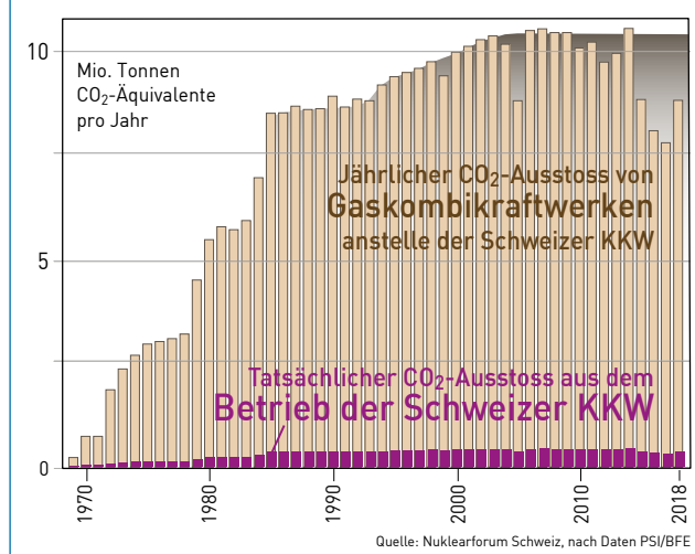
Abb. 2 Durch Schweizer Kernkraftwerke eingesparte CO 2 -Emissionen
